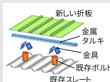
サドル工法 (間接固定工法の一つ) ▲
